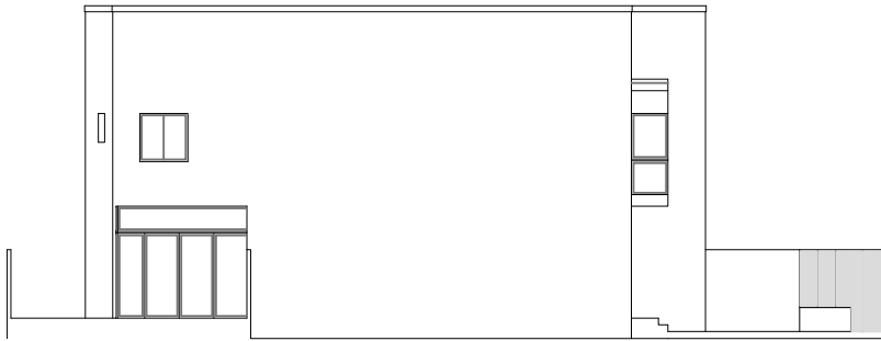
ALZADO ESTE
