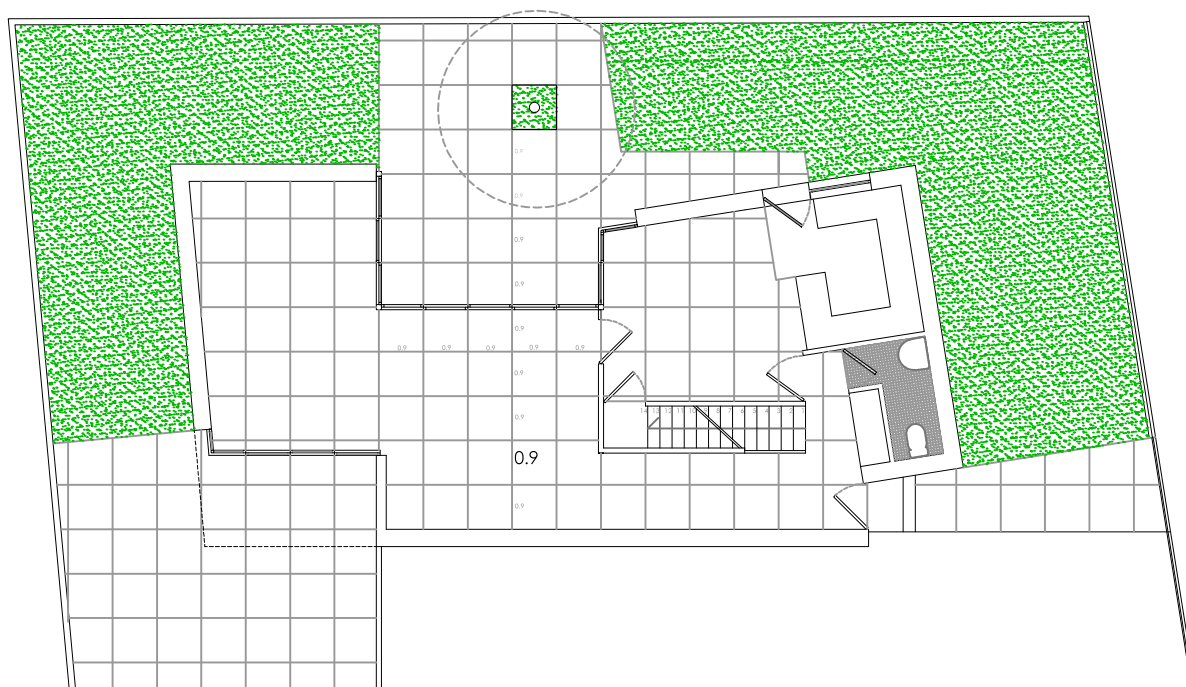
PLANTA BAJA-ACCESO
