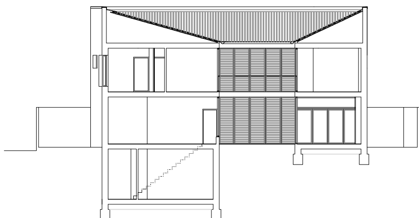
SECCION D-D'
