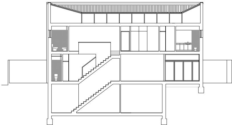
SECCION C-C'
