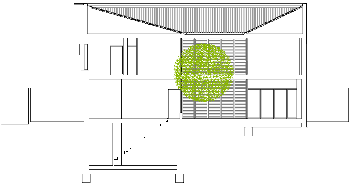
SECCION D-D'
