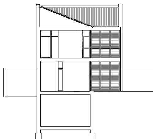
SECCION B-B'
